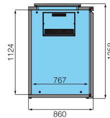
ADO 3H1 arrefecedor de detritos orgânicos waste disposal coolers refroidisseurs des déchets enfriadores de residuos
